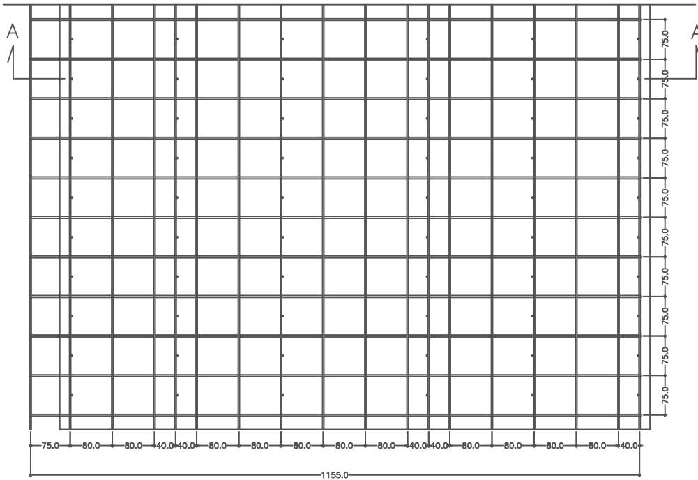
ИЗГЛЕД ПАНЕЛ
