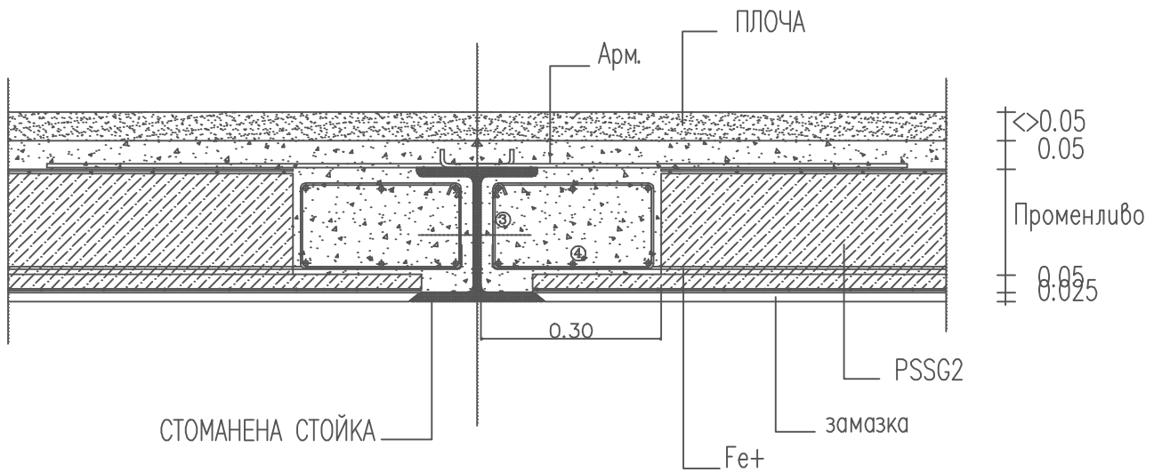
РАЗРЕЗ А-А
