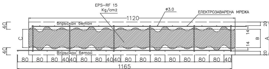
Единичен панел CS с приобвдигнат вълнов профил РАЗРЕЗ А-А
